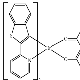
Btp 2 Ir(acac)
