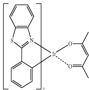
\text{Ir}(\text{BT})_2(\text{acac})
